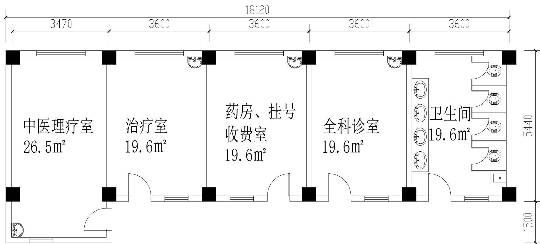
大铲岛社区健康服务站平面图 (套内)总面积: 104.9m 2
